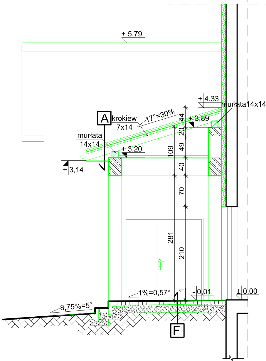
FRAGMENT PRZEKROJU D-D SKALA 1:50
