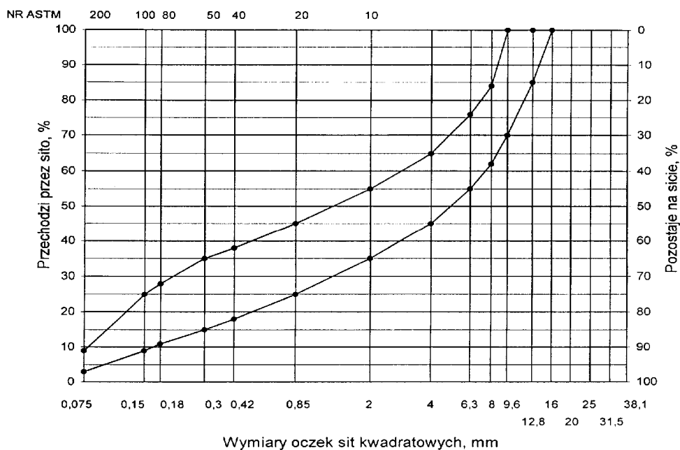
Rys. 10. Krzywe graniczne uziarnienia mieszanki mineralnej BA od 0 do 12,8 mm do warstwy wiążącej i wyrównawczej nawierzchni drogi o obciążeniu ruchem KR1 lub KR2
