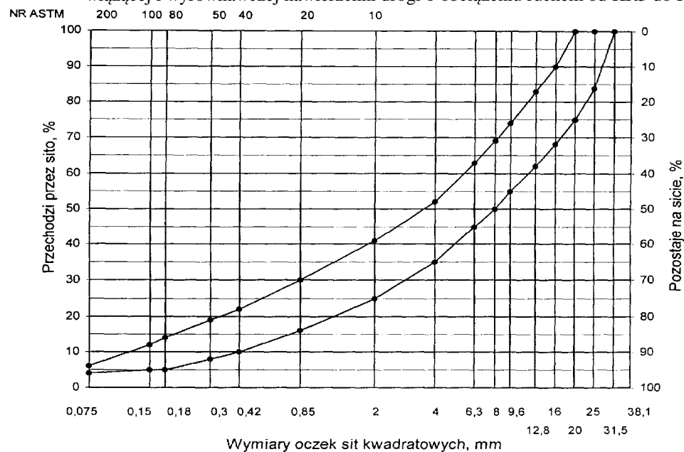
Rys. 11. Krzywe graniczne uziarnienia mieszanki mineralnej BA od 0 do 25 mm do warstwy wiążącej i wyrównawczej nawierzchni drogi o obciążeniu ruchem od KR3 do KR6
